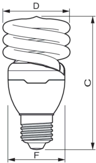
QSPIR-F 20W/865 E27 220-240V 50/60Hz
